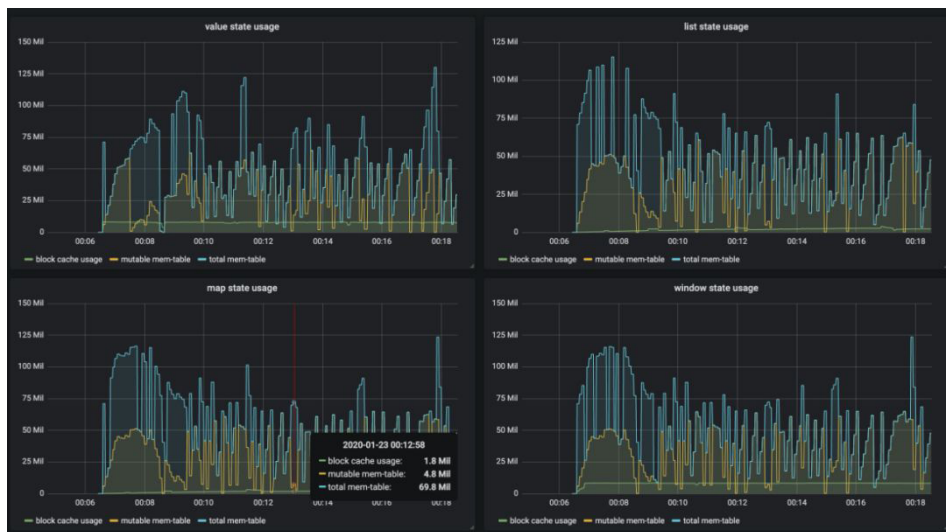
受控前的内存使用情况 (share-slot)
