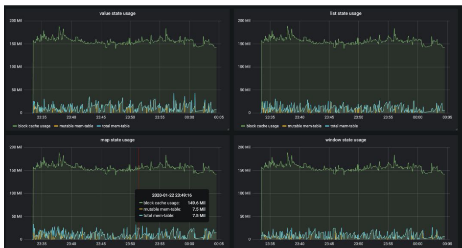
受控后的内存使用情况 (share-slot)
